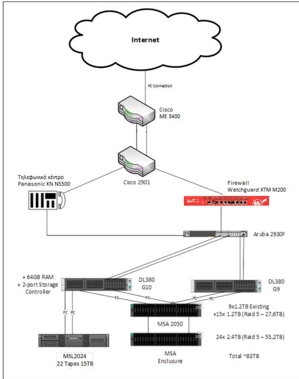
Σχήμα 2. Υποδομή μηχανογραφικών συστημάτων της ΕΦ μετά την αναβάθμιση
