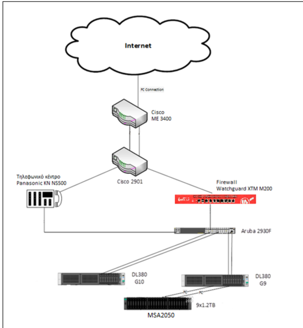
Σχήμα 1. Υφιστάμενη υποδομή της μηχανογραφικής υποδομής της ΕΦ
