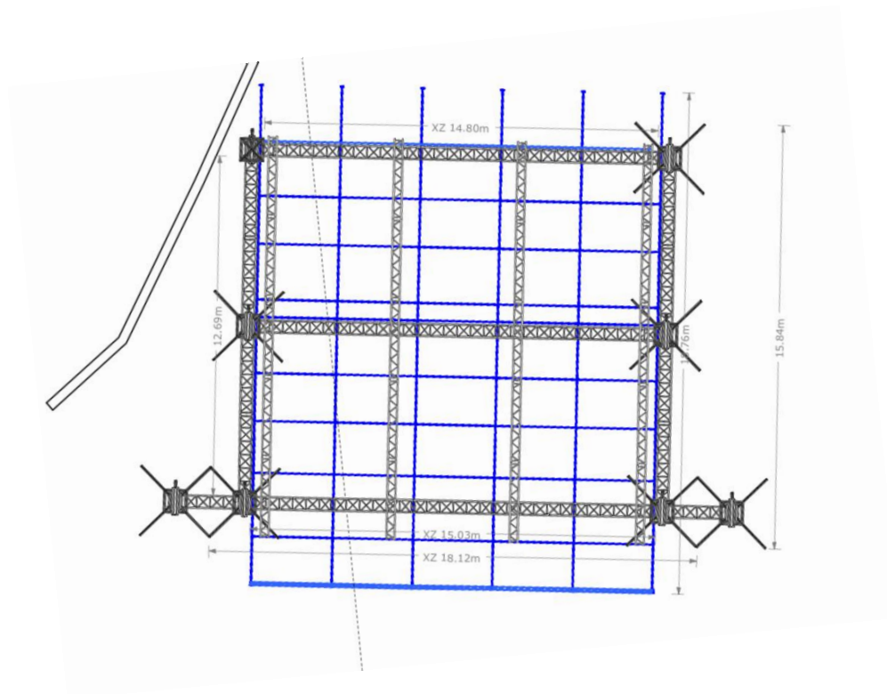
Ενδεικτικό σχέδιο χωροδικτύωματος Λυκαβηττού
